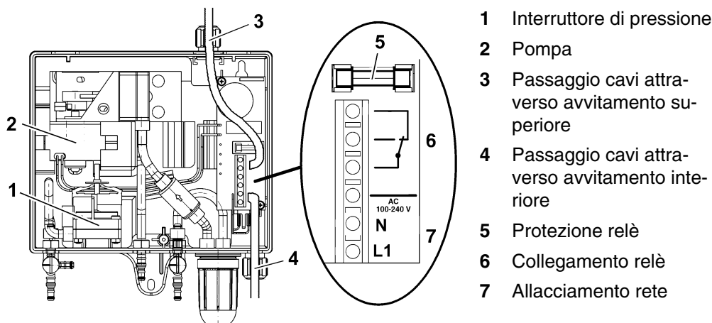
Fig. 5: Allacciamento elettrico
